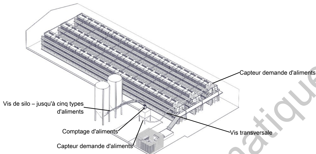
Figure 6: Schéma du système d'alimentation des poules dans un système de cage.
